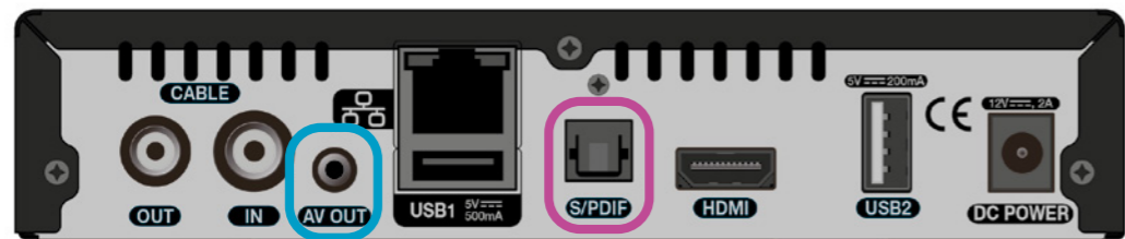
schemat podłączeń audio dla Odbiornika ARC1010YR / ARC1011YR
